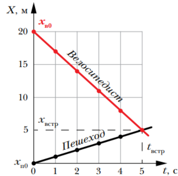
Рис. 21 Точка пересечения графиков движения пешехода и велосипедиста является точкой их встречи. Она произошла через 5 с после начала движения
