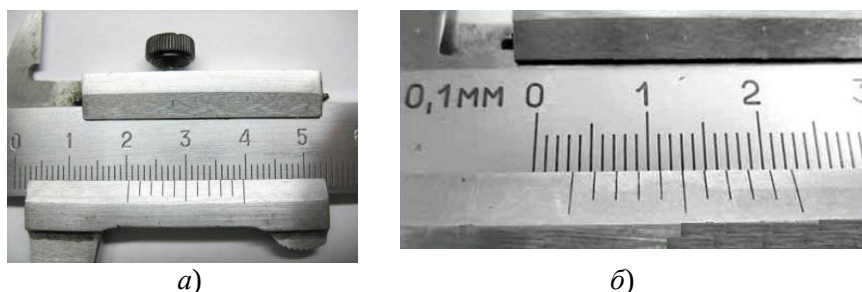
Рис. 11. Примеры измерения с помощью штангенциркуля.
